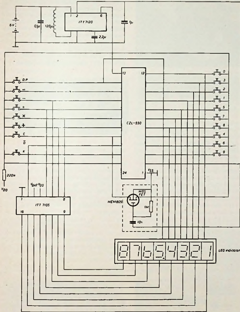
Fig. 4. Calculator met geïntegreerde klokimpuls-generator en automatisch resetcircuit bij het inschakelen.
